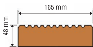
Schnitt Stegbohle
