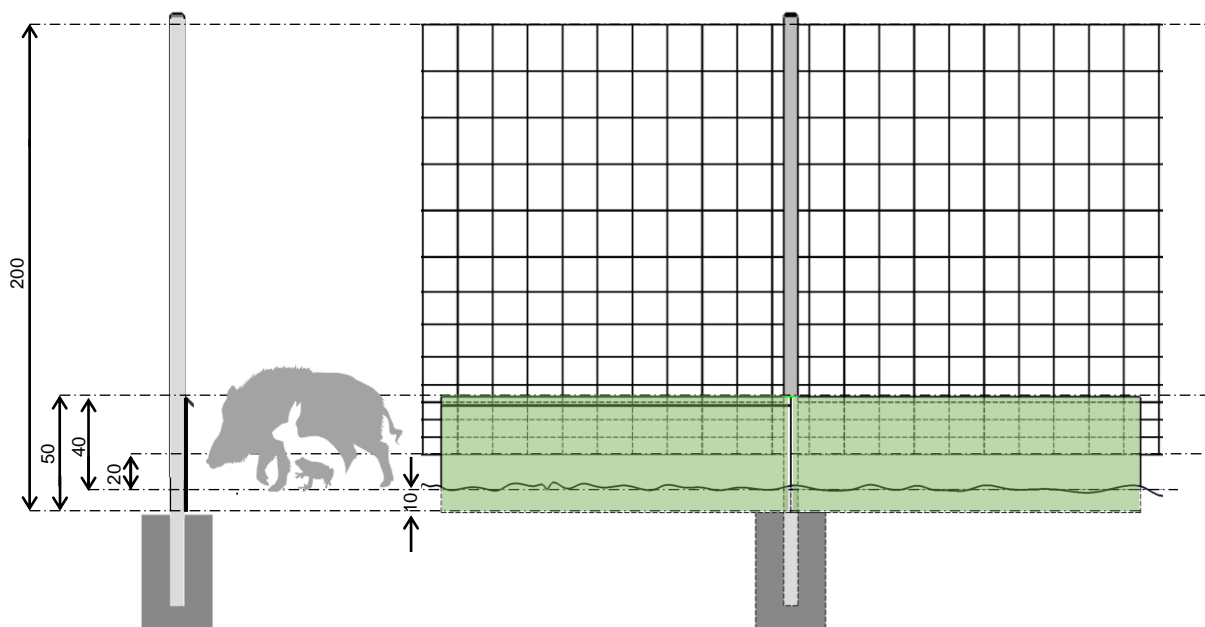
Typ A - mit molchsicherer Schutzkante
